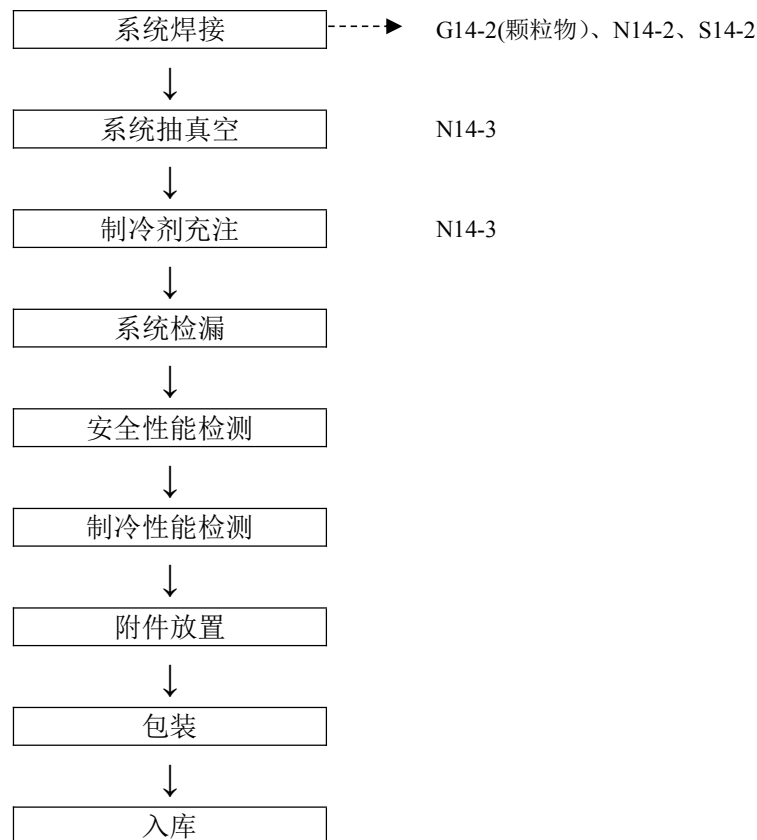
图 3.7-16 总装工艺流程图
