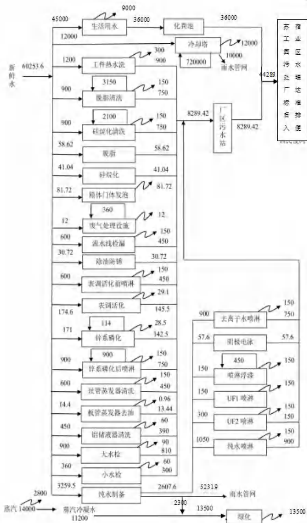
图3.8-1 水平衡图
