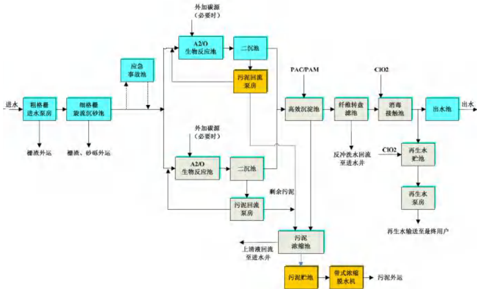
图6.2-8 苏州宿迁工业园区污水处理厂工艺流程
