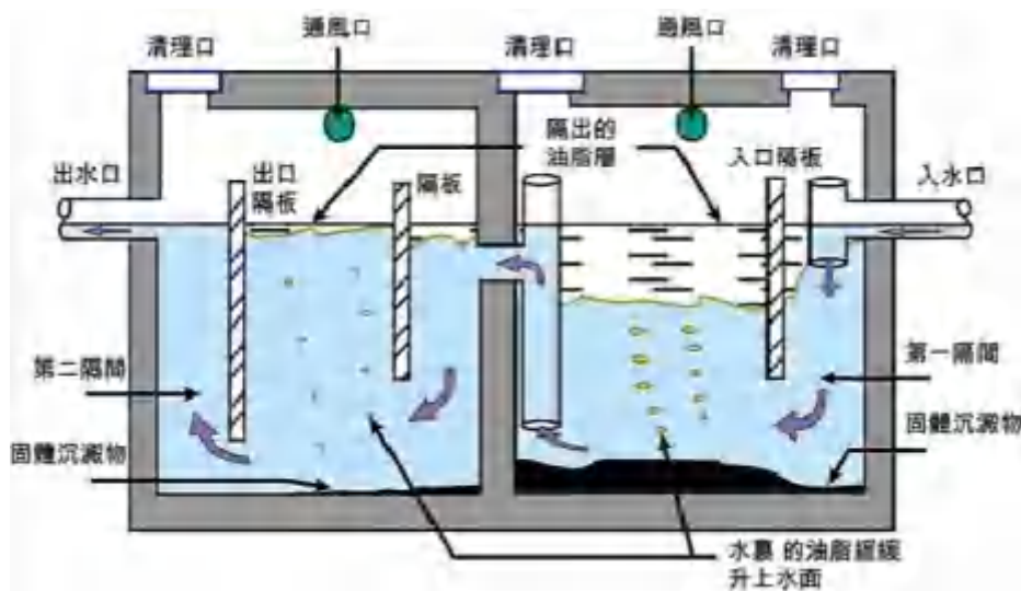
隔油池结构及工艺示例图
