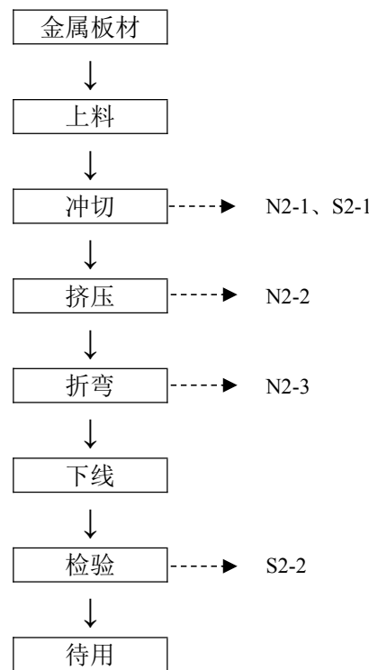
图3.7-4 小钣金成型工艺流程图
