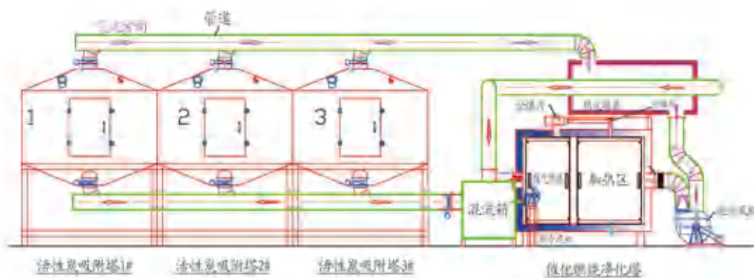
图6.2-2 催化燃烧结构图
