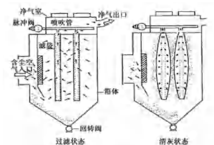
图6.2-1 脉冲喷吹布袋除尘器处理工艺示例图
