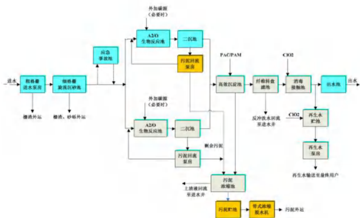
图4.3-1 污水处理厂工艺流程图
