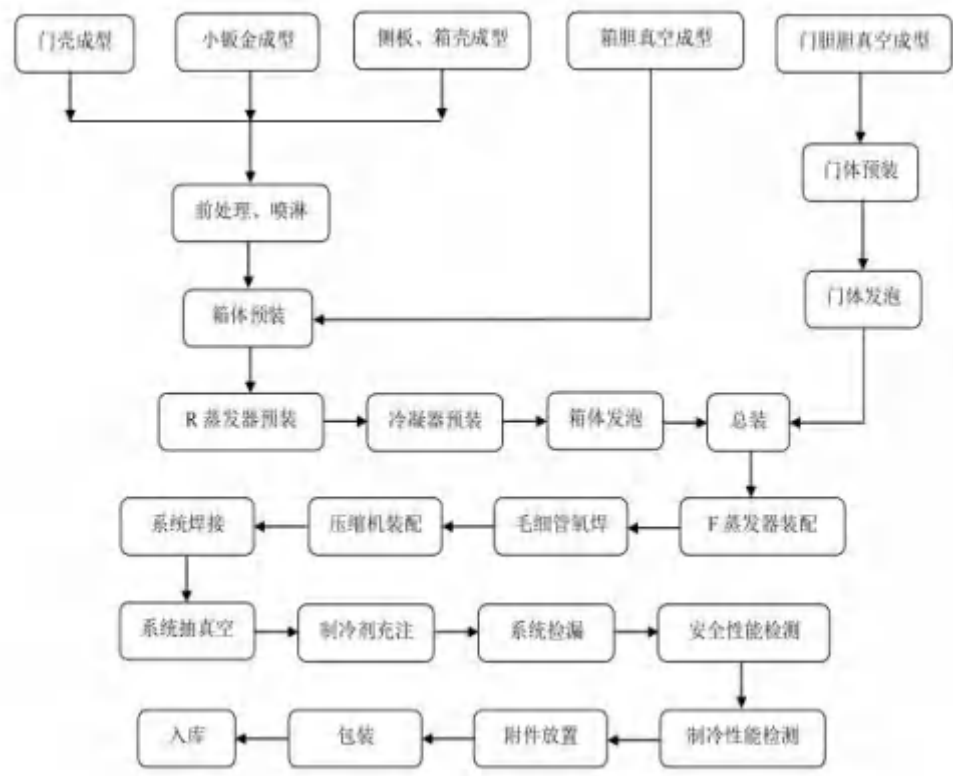
图3.7-2 生产工艺总流程图
