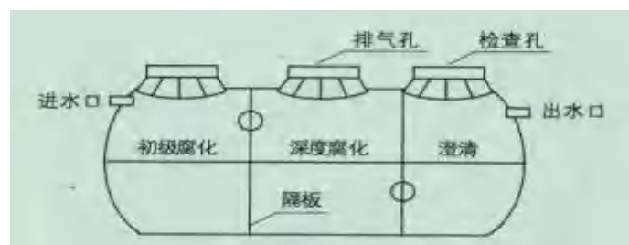
图6.2-7 化粪池工艺流程图
