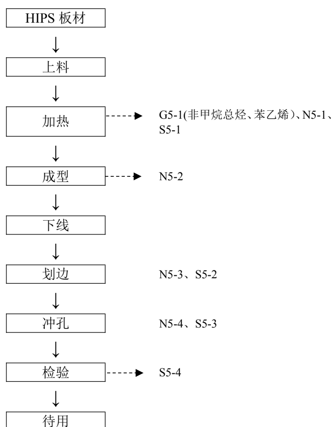
图3.7-7 箱壳成型工艺流程图
