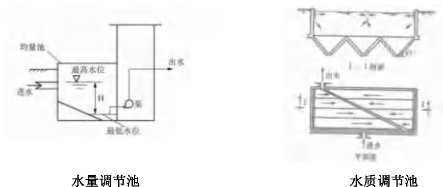
图6.2-4 水量水质调节池结构图
