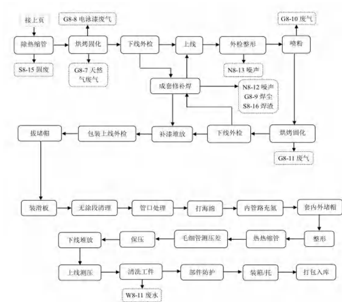
图3.7-10 丝管蒸发器生产工艺流程图
