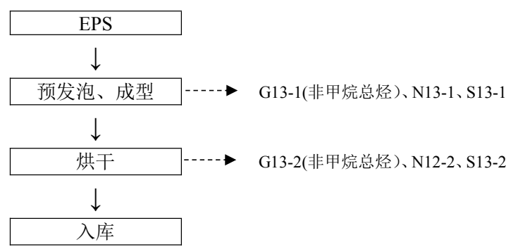
图3.7-15 EPS 发泡工艺流程图
