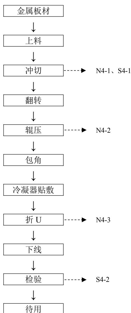
图3.7-6 箱壳成型工艺流程图
