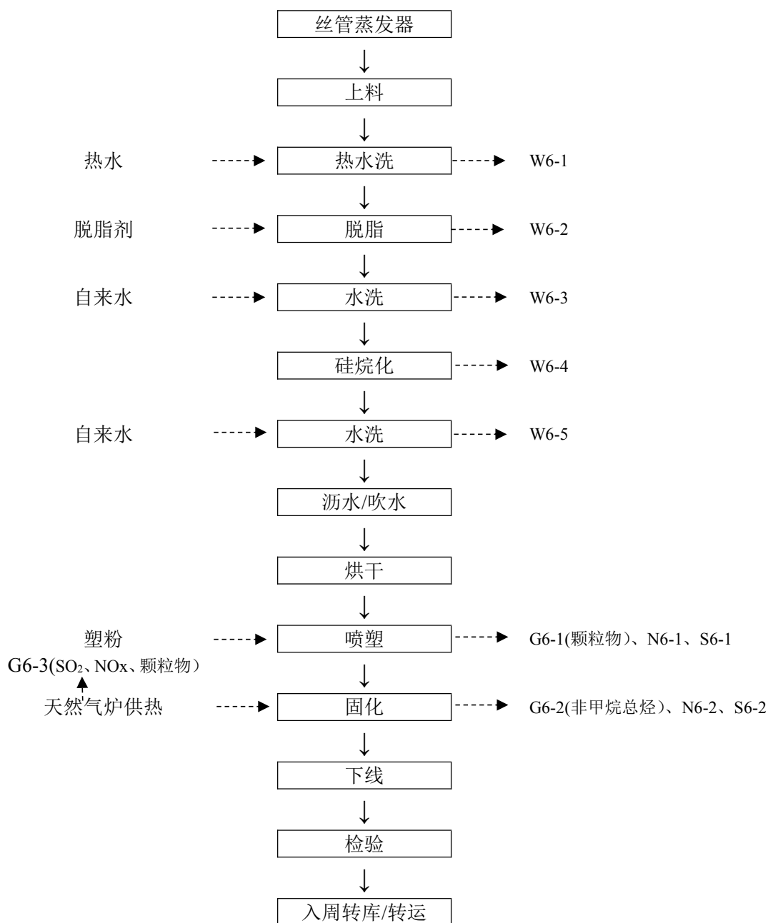
图3.7-8 磷化喷涂工艺流程图
