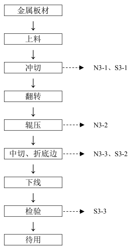
图3.7-5 侧板成型工艺流程图
