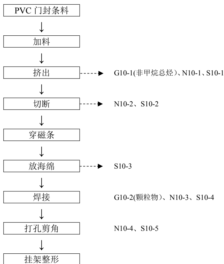
3.7-12 门封条 生产工艺流程图
