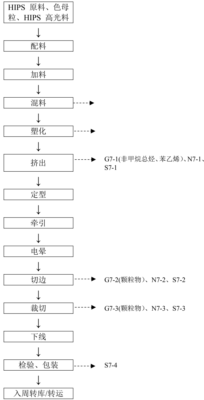
图 3.7-9 挤板工艺流程图
